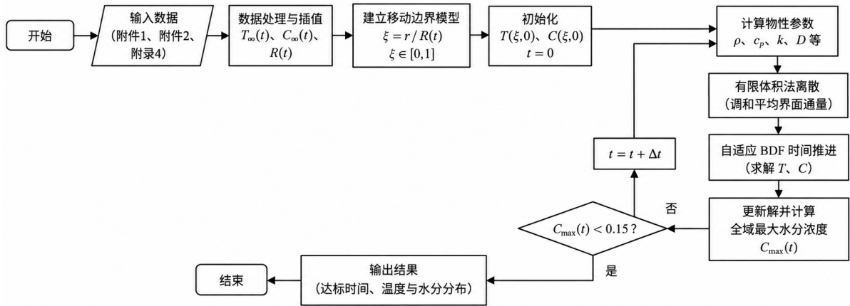
图 7 基于物质坐标变换与自适应 BDF 的问题四数值求解流程
