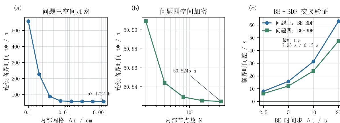
图 10 空间离散与时间积分的数值收敛及交叉验证结果
