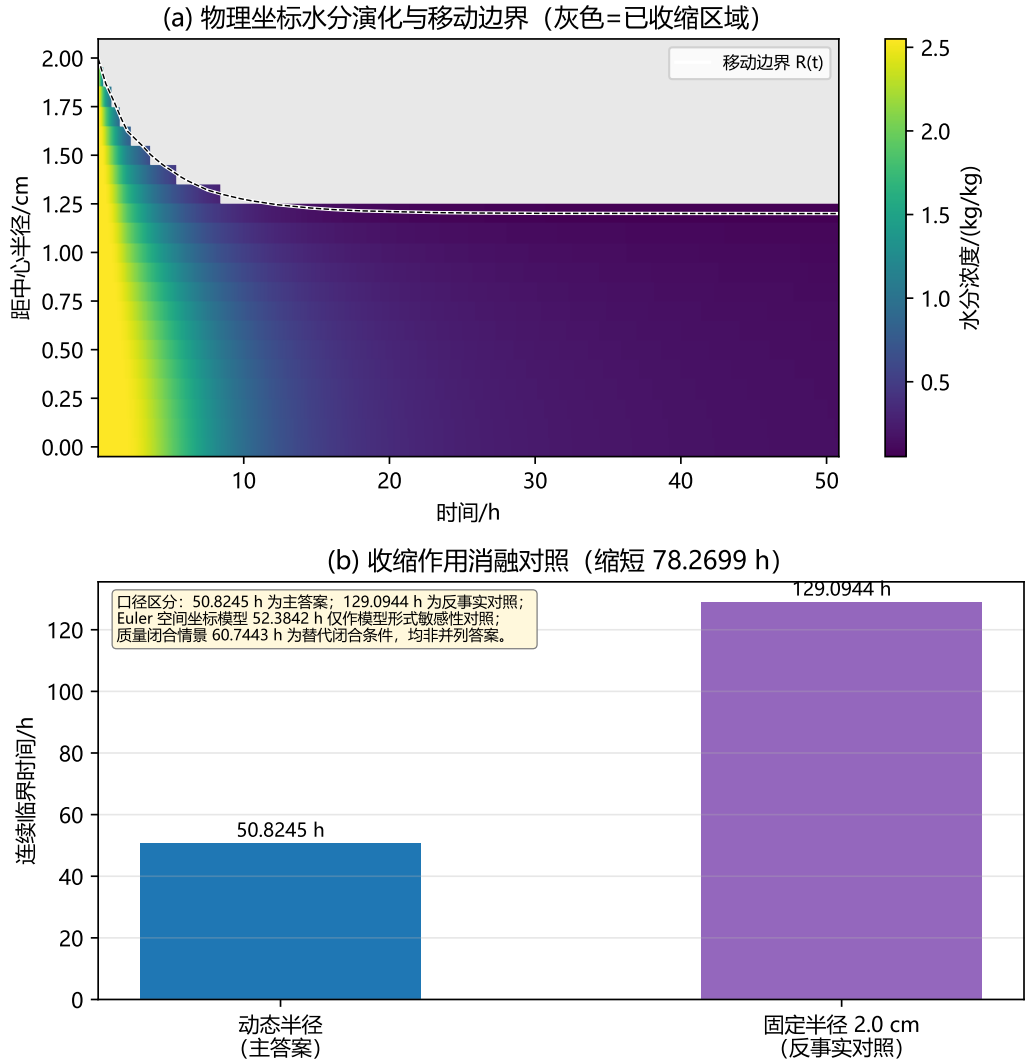
图 8 半径收缩条件下水分浓度演化及收缩作用对照。(a) 物理坐标下水分浓度热力图，白色曲线为移动边界 R(t) ，灰色为已收缩退出的药材区域；(b) 相同附录 4 物性与边界条件下动态半径与固定半径 2.0 cm 的连续临界时间消融对照，图内方框给出各对照值与主答案的口径区分。
