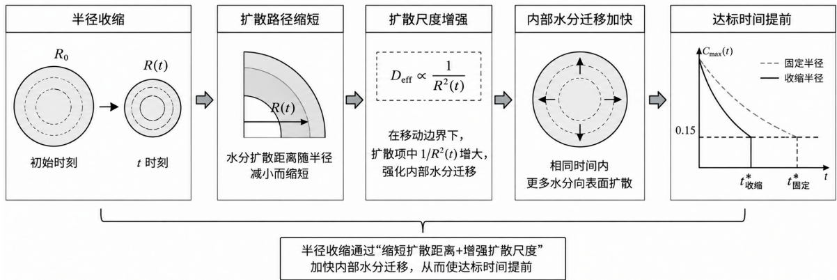
图 9 半径收缩促进内部水分迁移并缩短达标时间的作用机制
