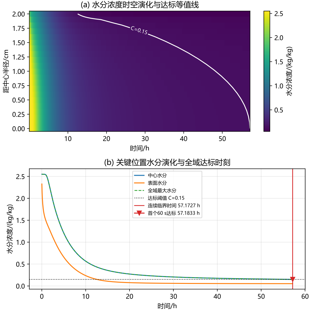
图 4 固定半径条件下水分浓度演化及全域达标时刻。(a) 水分浓度时空热力图，白色曲线为 C = 0.15 \text{ kg/kg} 达标等值线；(b) 中心、表面与全域最大水分随时间演化，水平点线为达标阈值，竖线与三角标记分别给出连续临界时间与首个 60 s 达标时刻。
