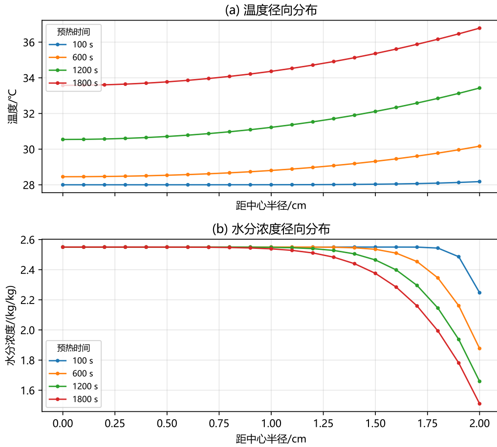
图1 问题一预热阶段药材温度与水分浓度的径向演化。(a) 100 s、600 s、1200 s 与 1800 s 的温度径向分布；(b) 对应时刻的水分浓度径向分布。温度自中心向表面升高并随时间整体上移；水分浓度在 1800 s 内仅近表面区域明显下降，中心保持初值，表明传热明显快于水分扩散。
