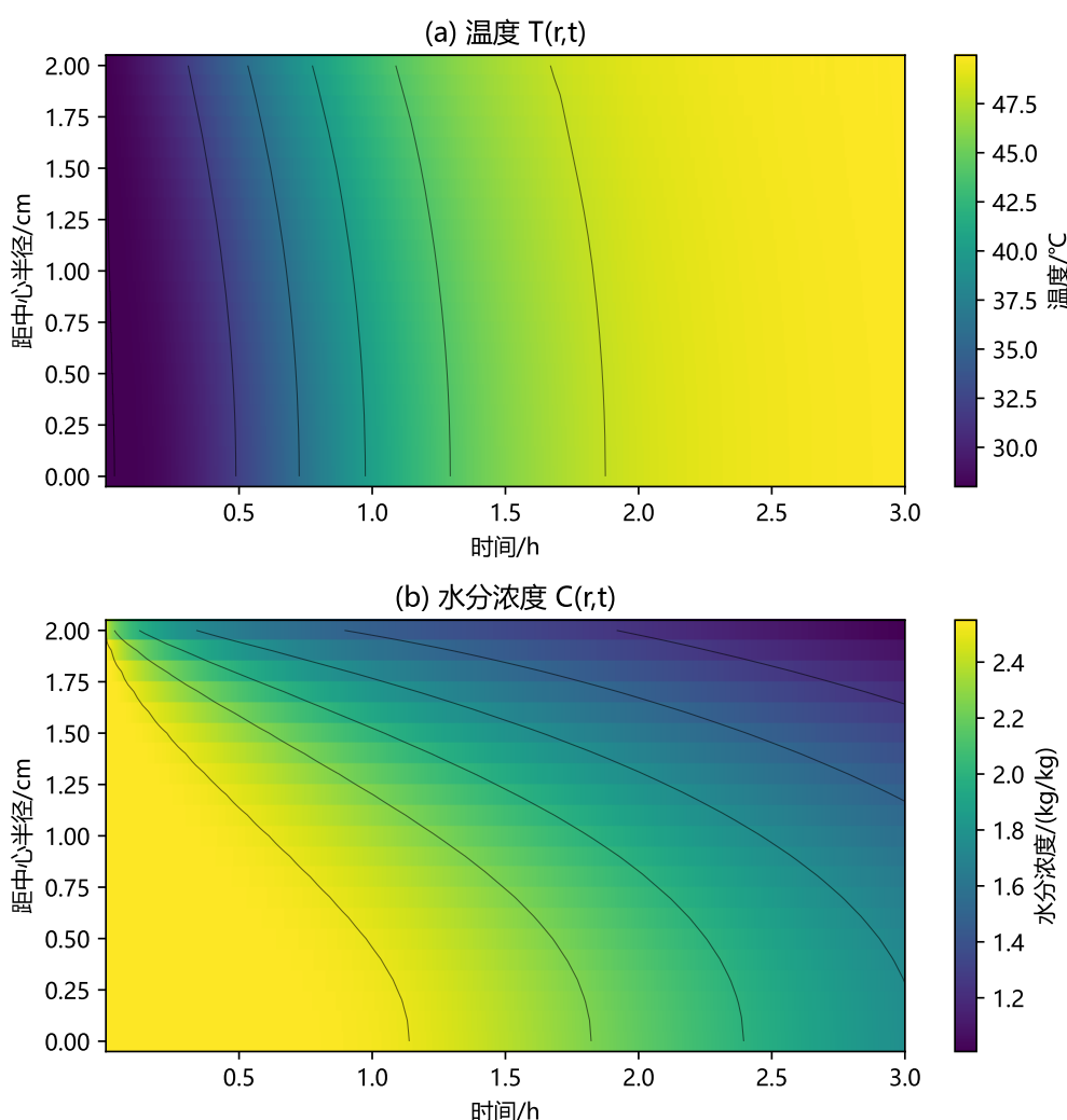
图3 变物性热湿耦合条件下温度与水分浓度的时空演化。(a) 温度 T(r,t) ; (b) 水分浓度 C(r,t) ; 黑色细线为等值线。温度场约 2h 内接近烘房温度、径向梯度消失; 水分场在整个 3h 内保持明显径向梯度, 说明恒温干燥阶段受内部水分扩散控制。
