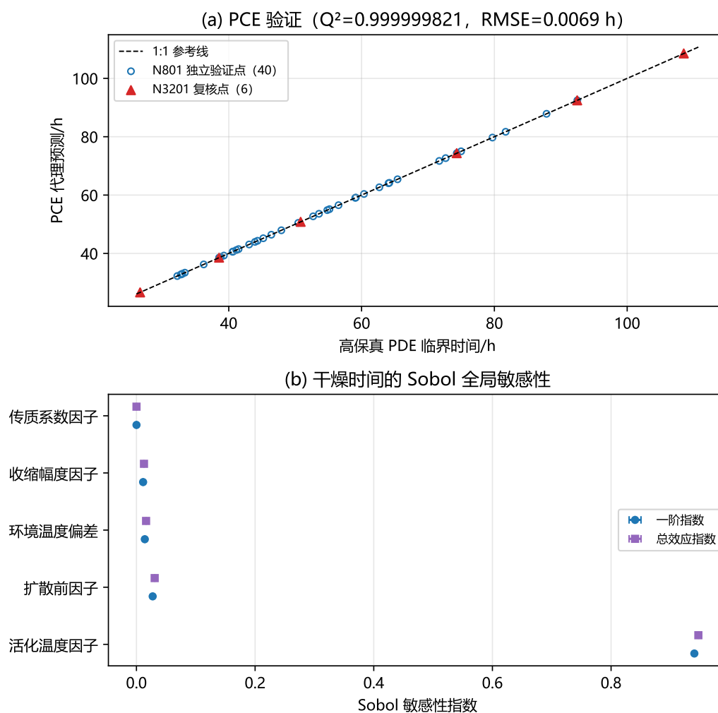
图 6 问题四代理模型验证与全局敏感性。(a) 4 阶多项式混沌代理预测与高保真 PDE 临界时间的对比，圆点为 40 个独立验证样本，三角为 6 个 N = 3201 复核样本；(b) 筛选后 5 个参数对干燥时间的 Sobol 一阶与总效应指数，误差棒为残差 bootstrap 的代理系数 95% 区间，不具有统计置信区间含义。
