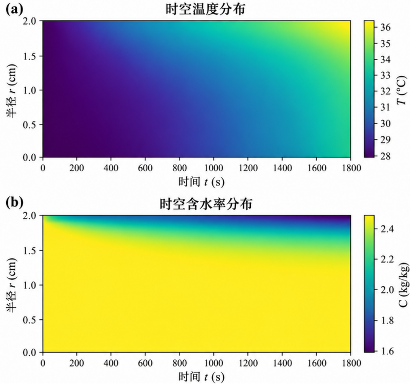
图2 预热平衡阶段（0–1800s）药材内部温度场与含水率场沿径向位置的时空演化特征。子图(a)展示温度分布，子图(b)展示含水率分布。
