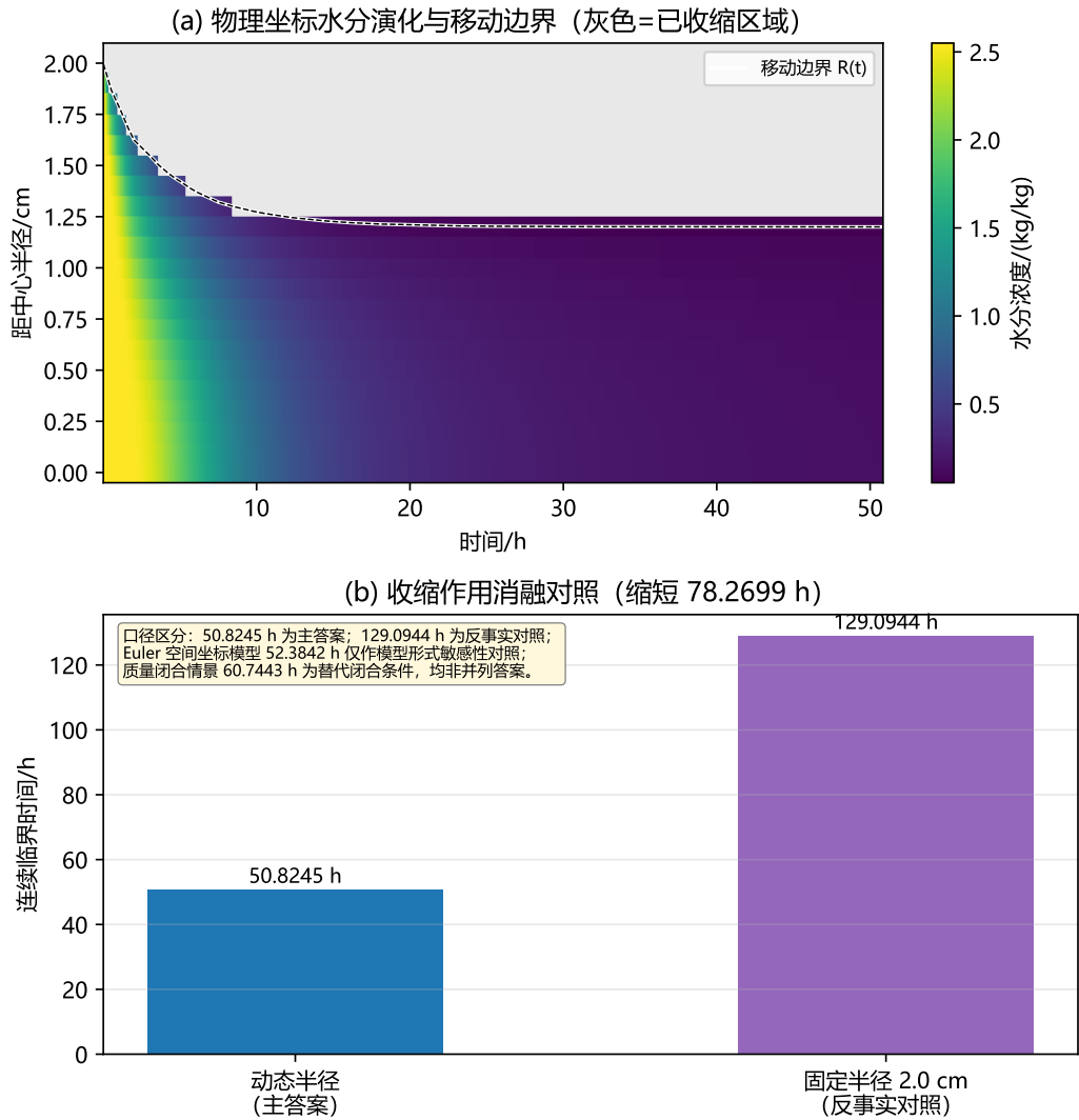
图 5 半径收缩条件下水分浓度演化及收缩作用对照。(a) 物理坐标下水分浓度热力图，白色曲线为移动边界 R(t) ，灰色为已收缩退出的药材区域；(b) 相同附录 4 物性与边界条件下动态半径与固定半径 2.0 cm 的连续临界时间消融对照，图内方框给出各对照值与主答案的口径区分。
