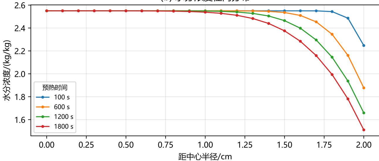
(b) 水分浓度径向分布
