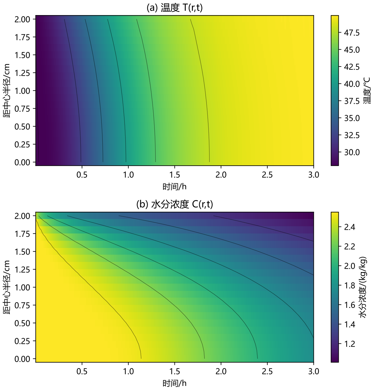
图3 变物性热湿耦合条件下温度与水分浓度的时空演化
