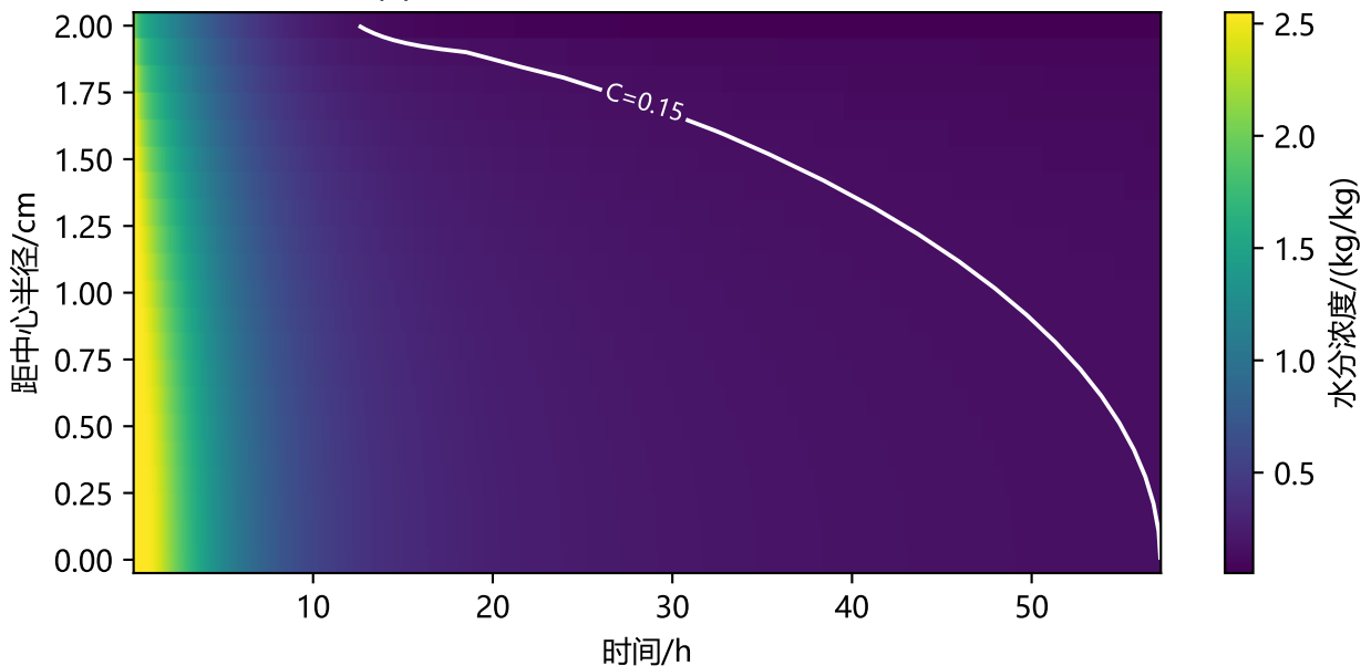
(b) 关键位置水分演化与全域达标时刻
