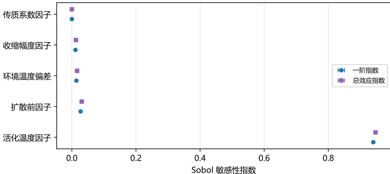
(b) 干燥时间的 Sobol 全局敏感性
