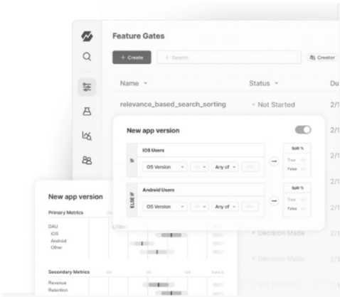
图10-5 默认开启的实验：功能开关 + 统计引擎 = 实验。把功能开关和实验做成同一个东西：功能开关负责按条件决定谁看到什么；统计引擎负责把用户随机分到不同的体验，并直接用已有的指标分析影响。这样，每次上线都自带实验结果
