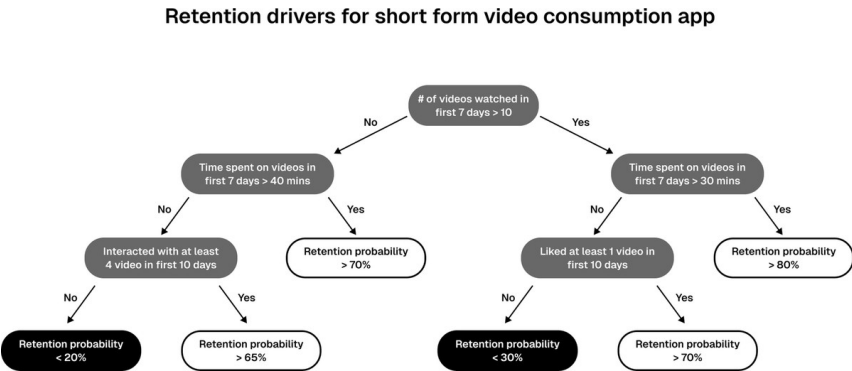
图2-14 短视频app的留存驱动因素决策树：第一层看头七天是否看了超过10个视频，再看看时长、互动和点赞，最右边一支（看了超过10个、时长超过30分钟）的留存概率超过80%
