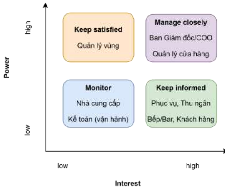
Hình 1.2 Power/Interest Grid
