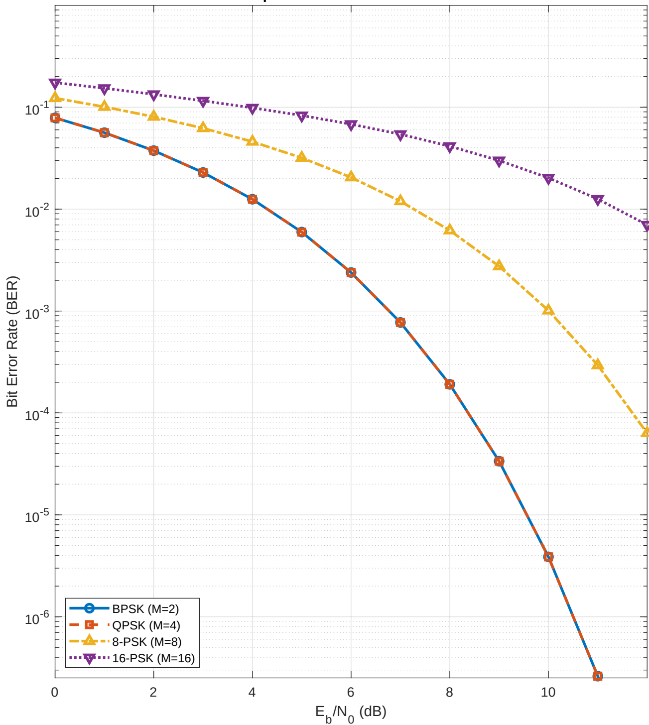
Confronto BER per diverse modulazioni M-PSK in AWGN
