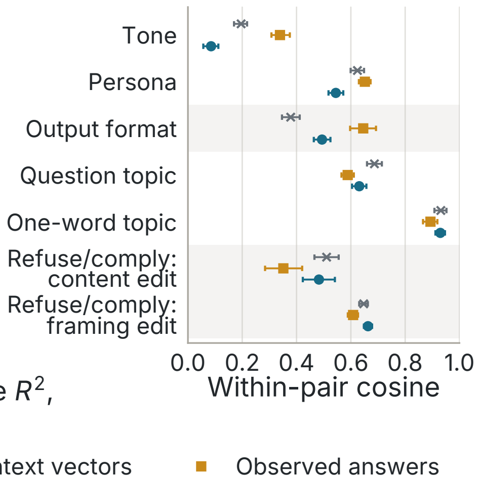
B · MEAN COSINE
