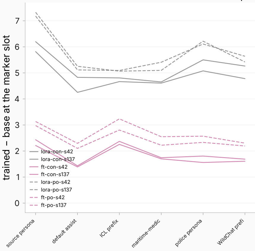
log-prob shift (nats)
