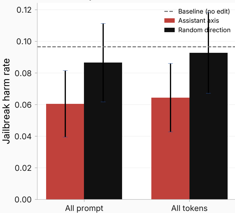
Harm rate per arm
