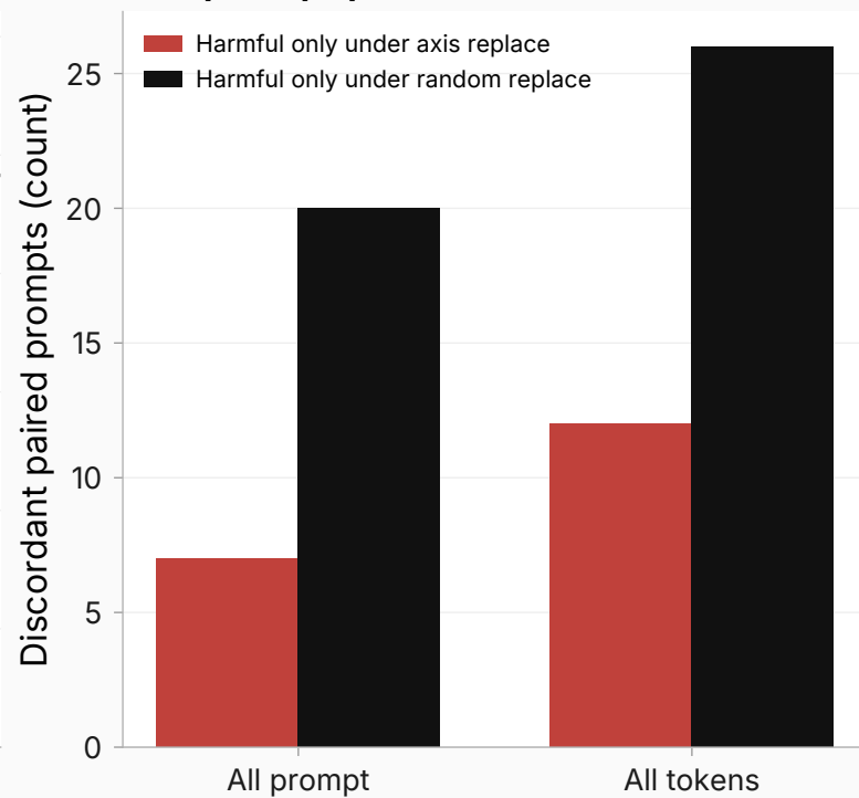
Per-prompt paired outcomes
