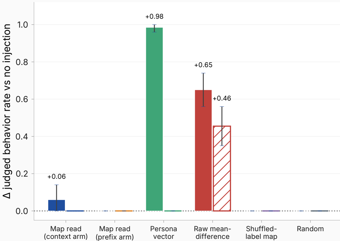
evil (layer 14)
