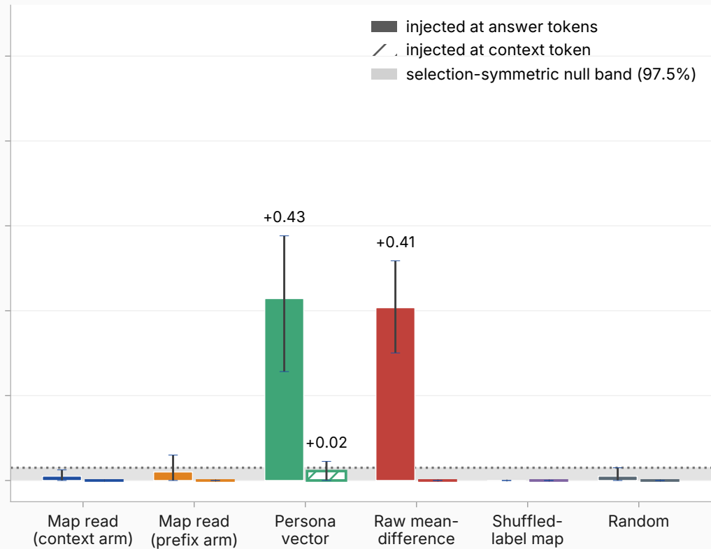
sycophancy (layer 18)
