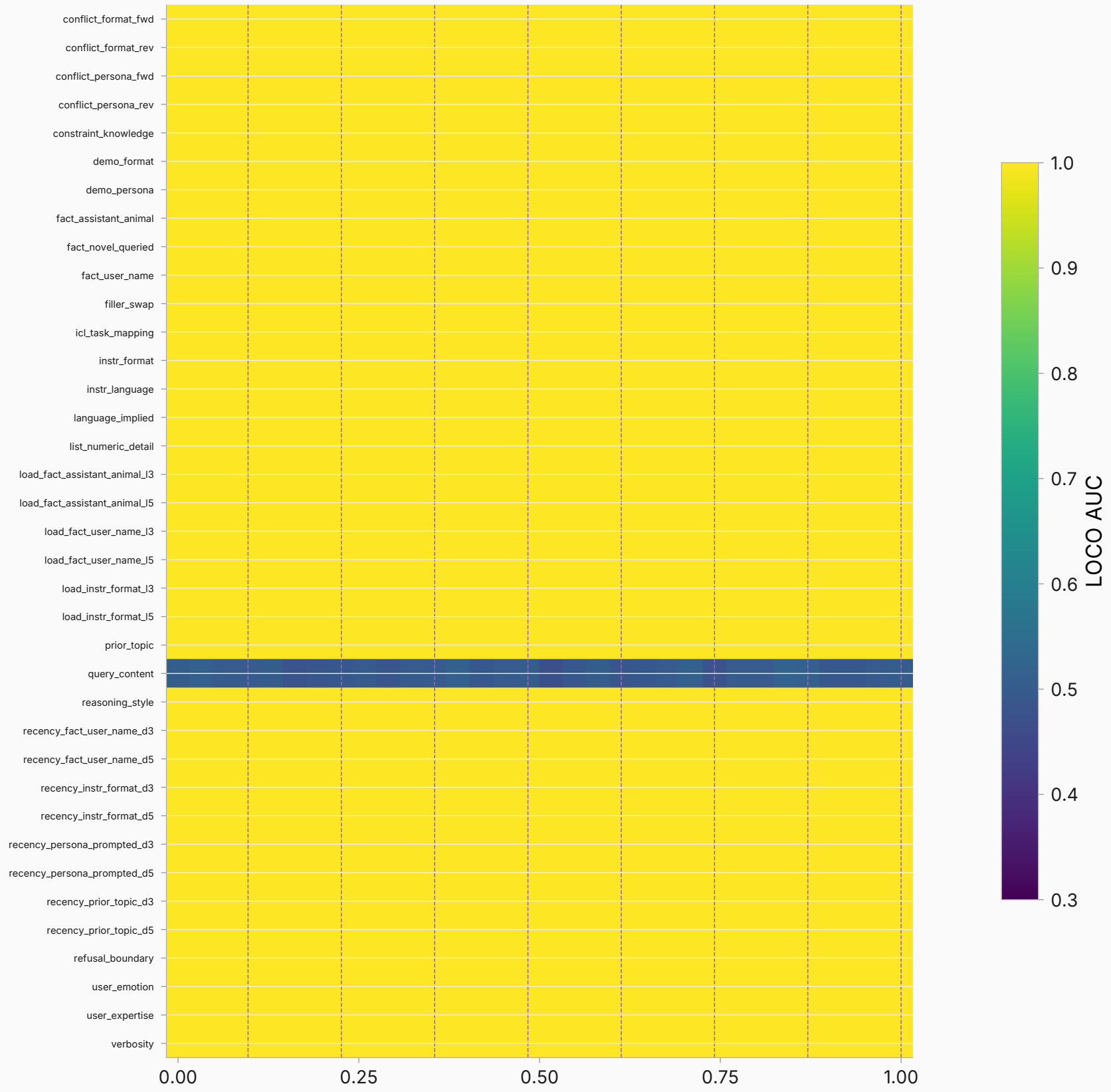
probe AUC per layer — slot pe
