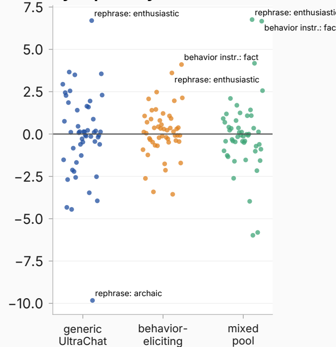
sycophancy
