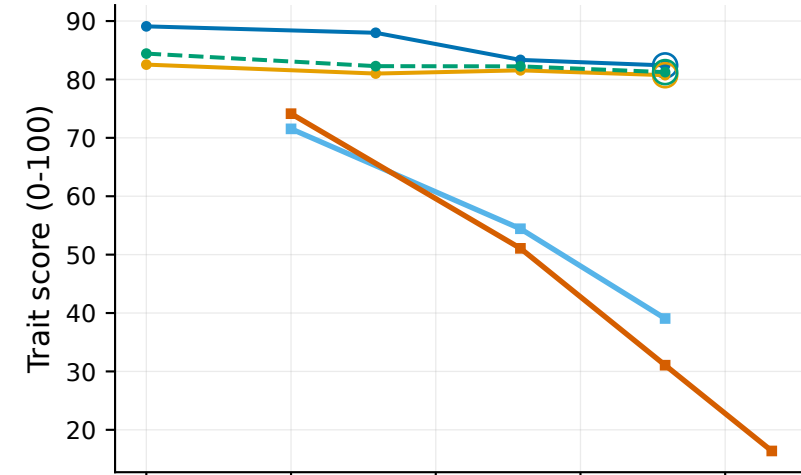
Evil II
