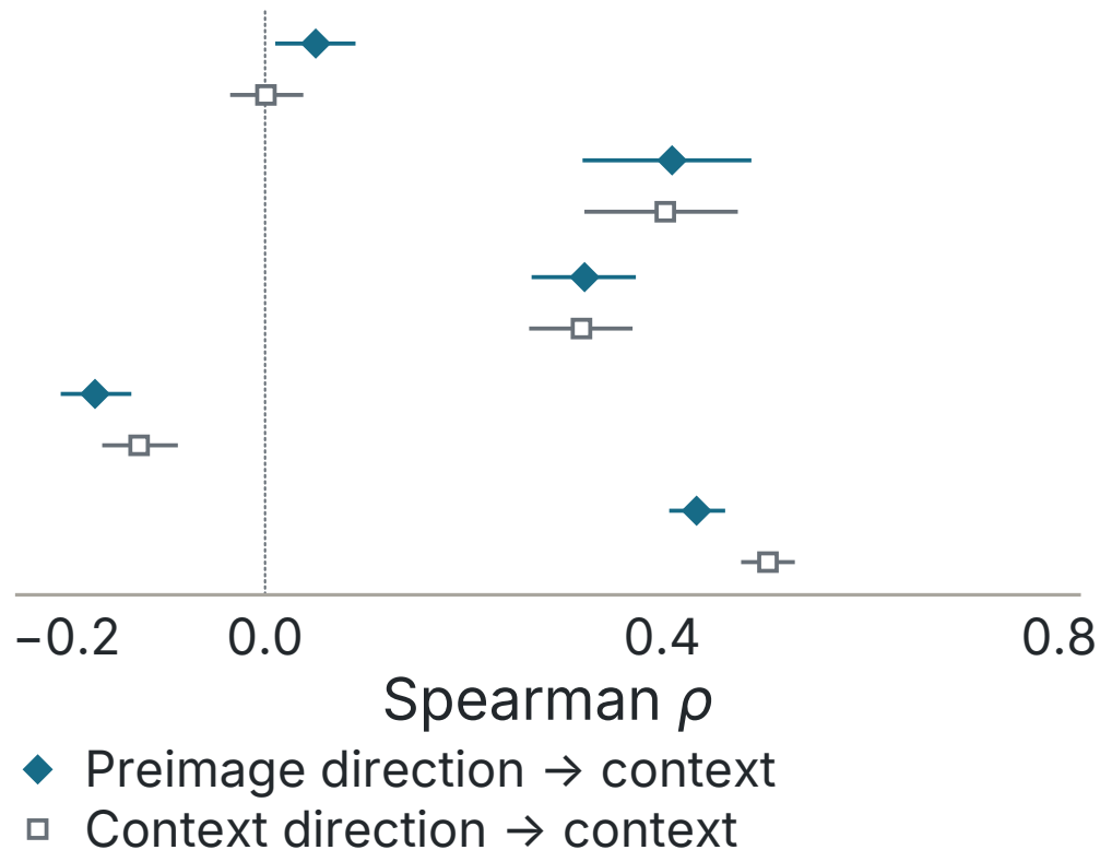
B · PREIMAGE DIRECTION
