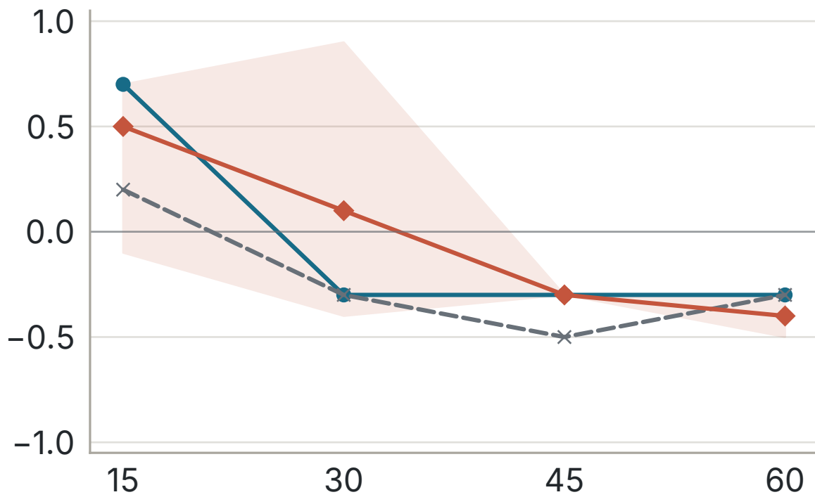
DeepSeek-V3.1-Base · HHH
