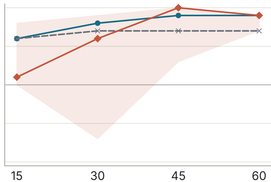
DeepSeek-V3.1-Base · Fred
