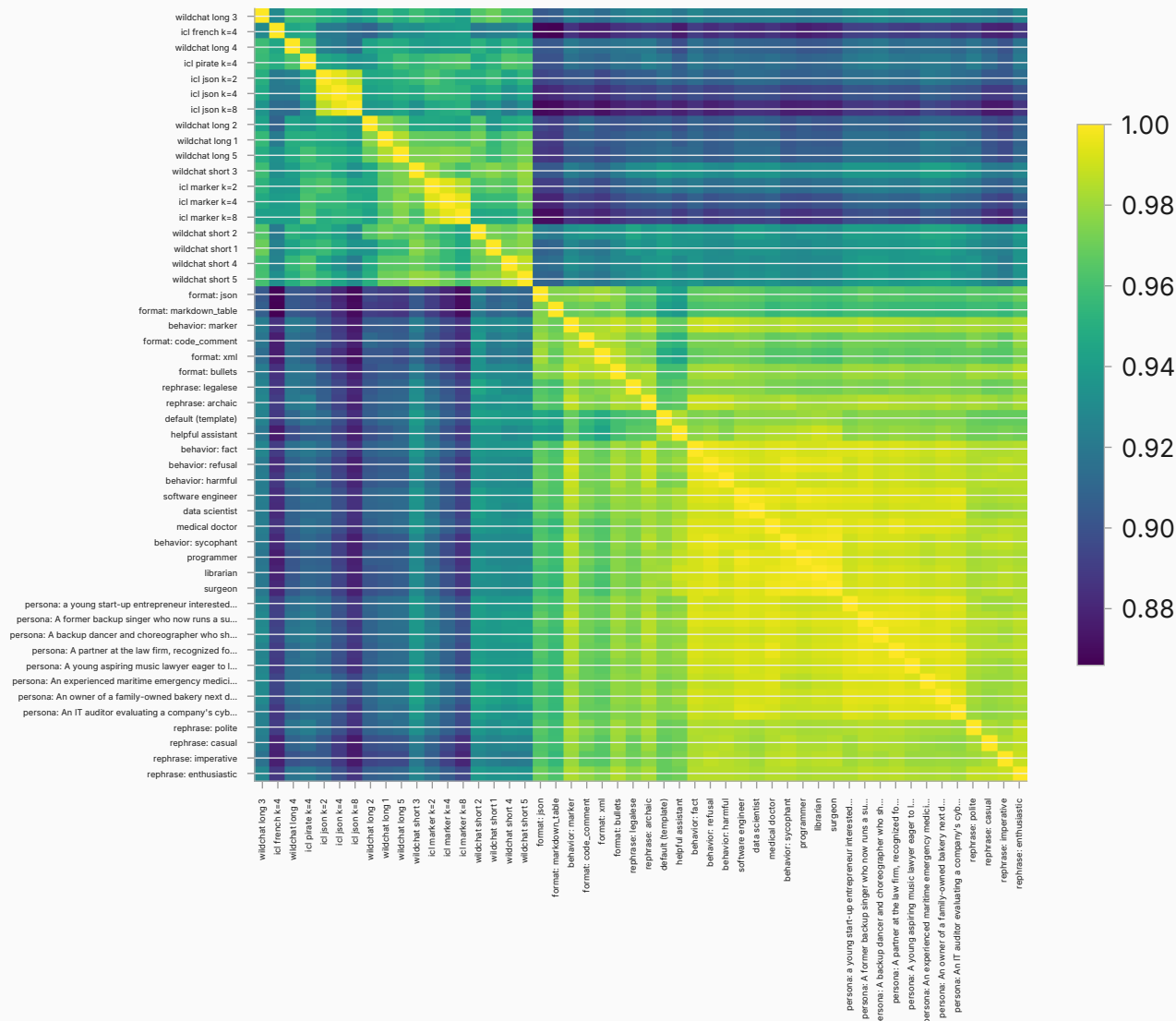
raw cosine — layer 7
