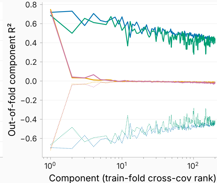
L18 (dotted = perm-null p95)
