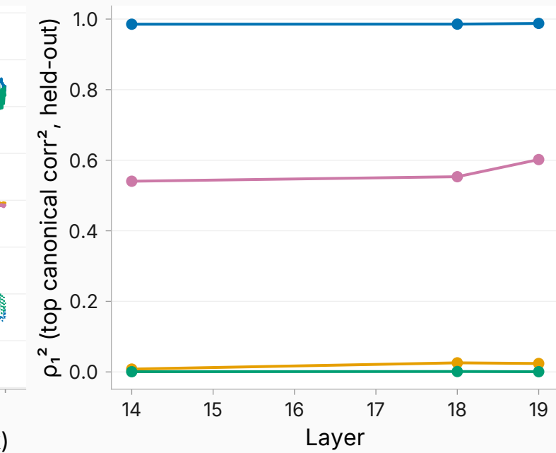
Linear-readout ceiling per layer
