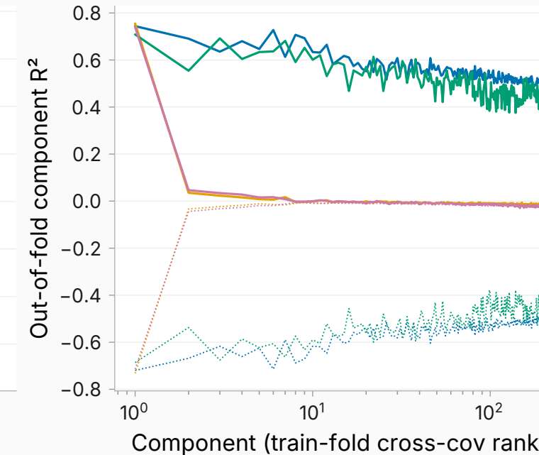
L19 (dotted = perm-null p95)
