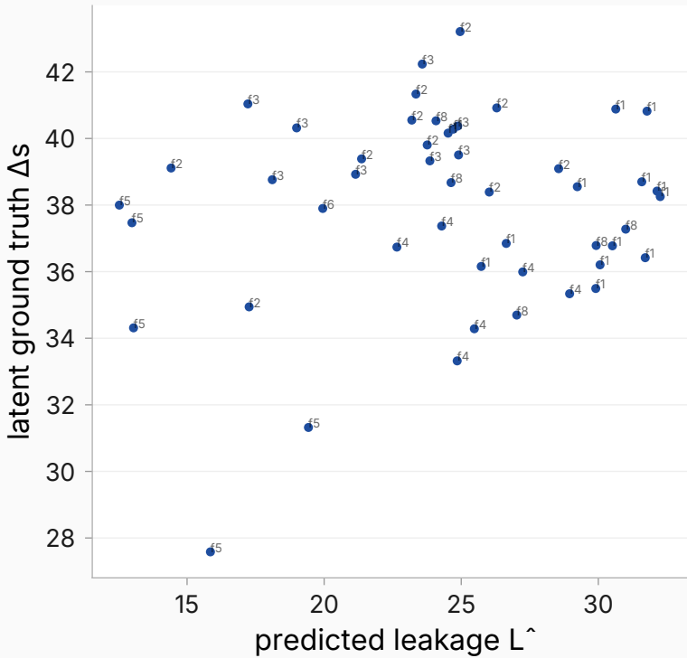
bm_default_posonly_d2_seed42 ( \rho=-0.065 )
