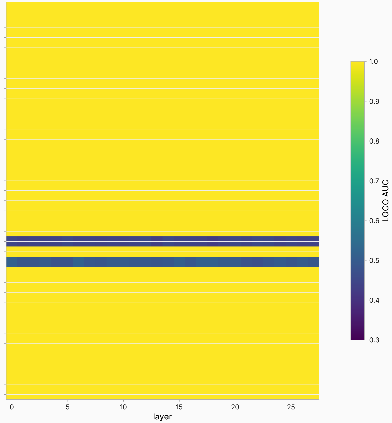
probe AUC per layer — slot pe
