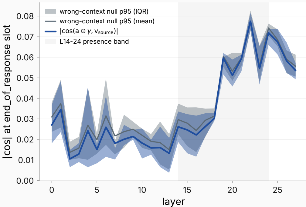
(a) Read arm — q_proj
