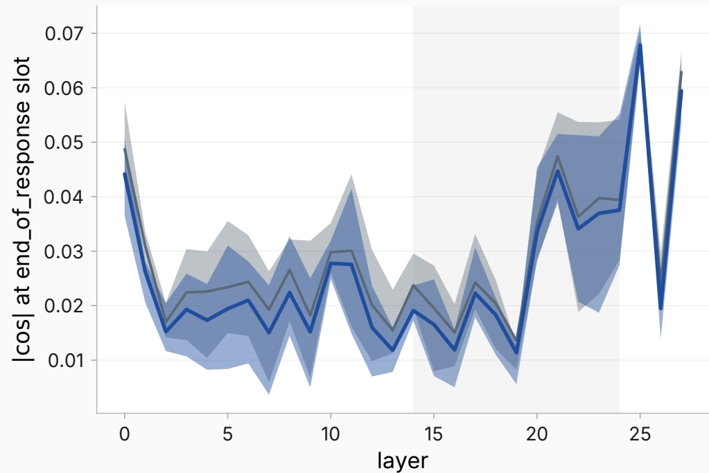
(b) Read arm — v_proj
