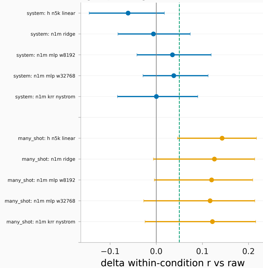
sycophancy
