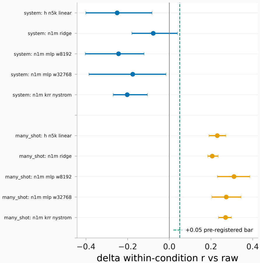
evil
