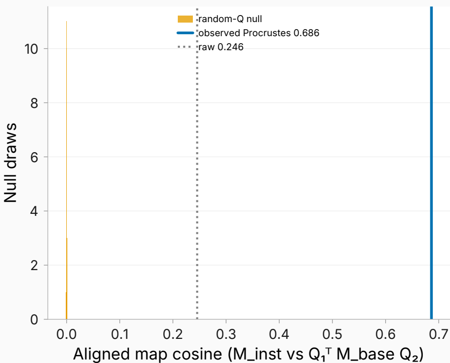
L19 Procrustes-cosine chance reference
