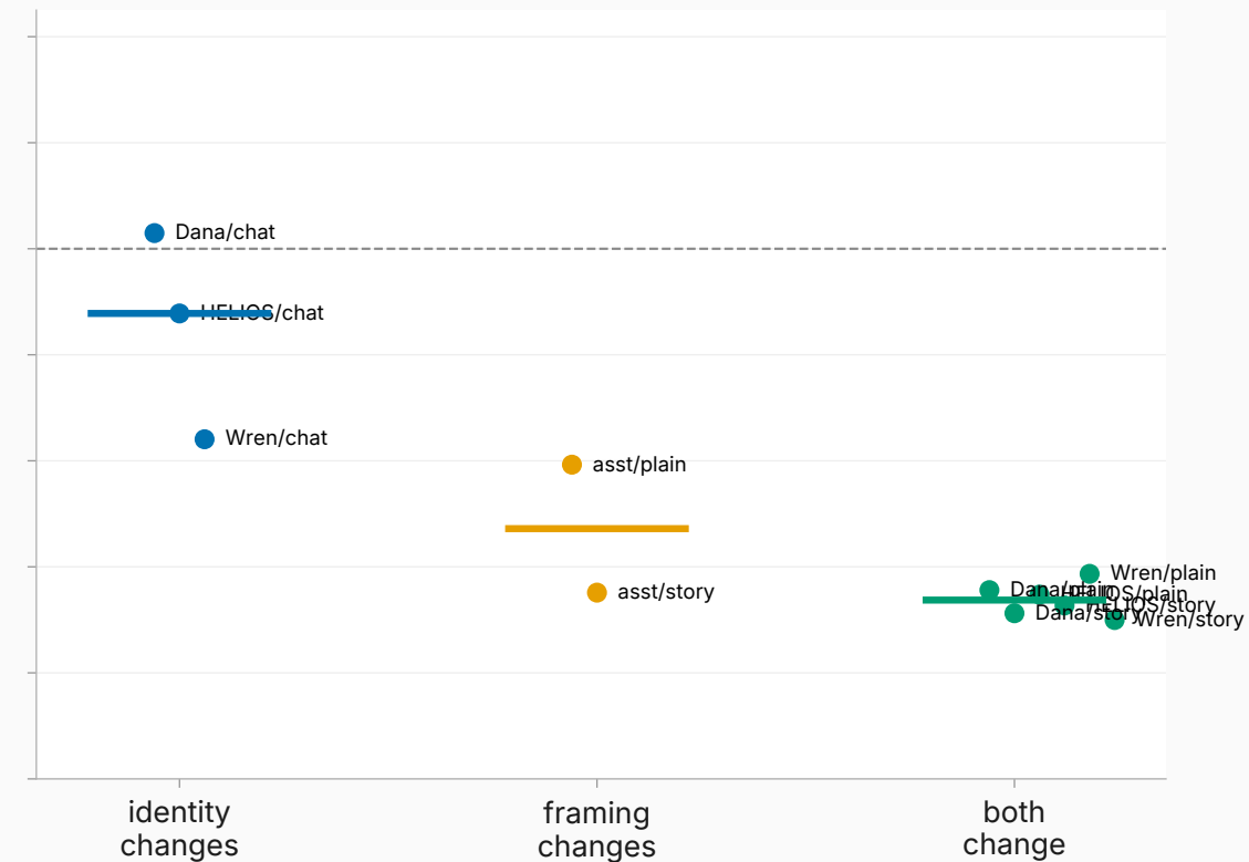
prefix arm
