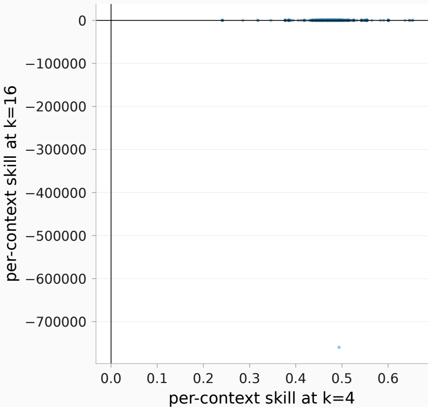
rollout skill per context (emb)
