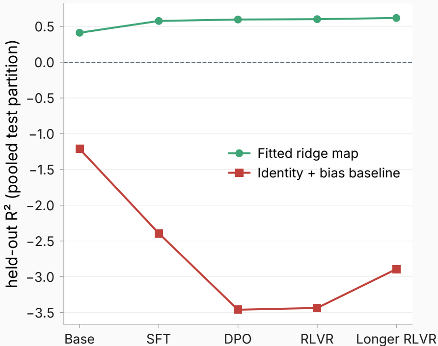
Held-out R^2 , layer 30
