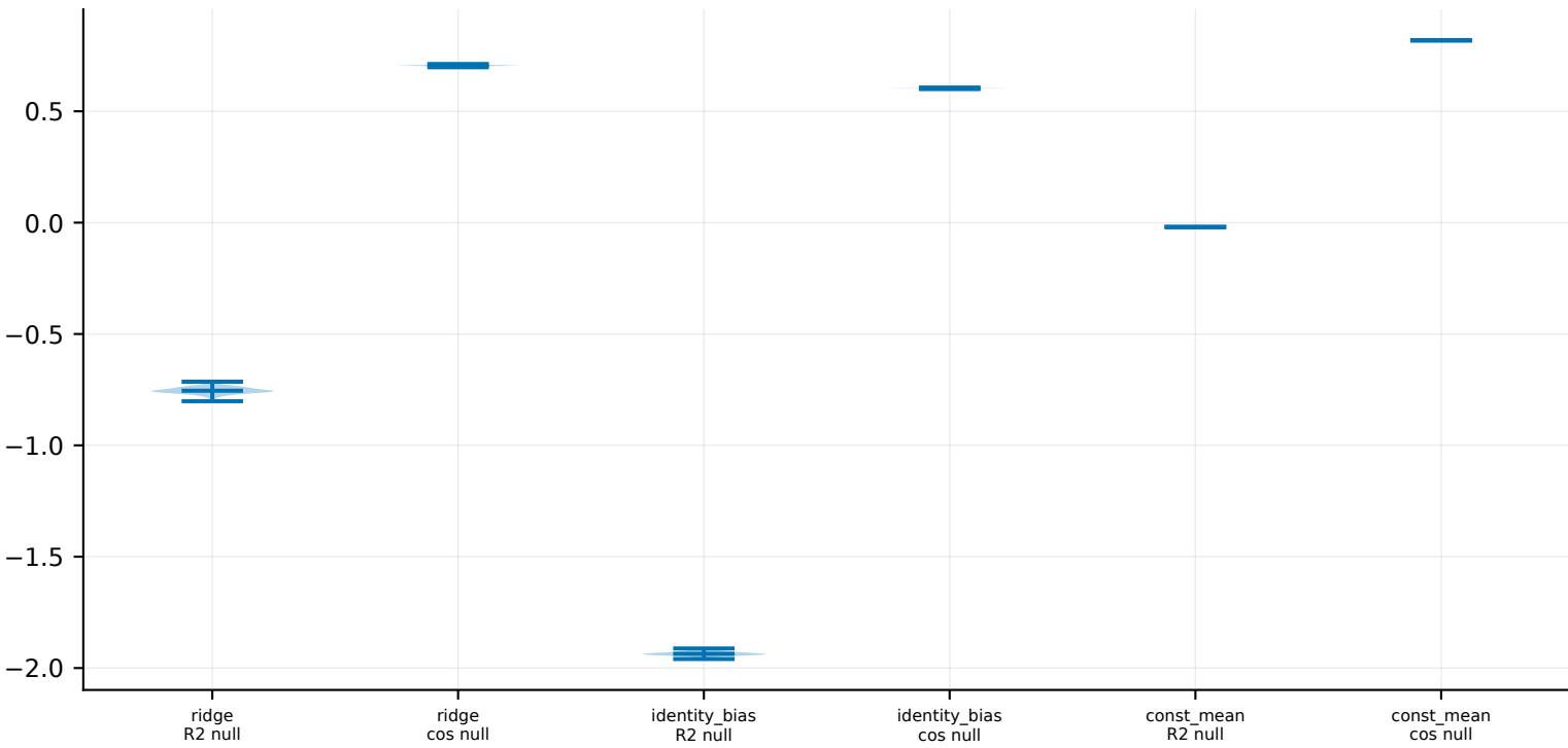
wc shuffled-pair null distributions (K=200)
