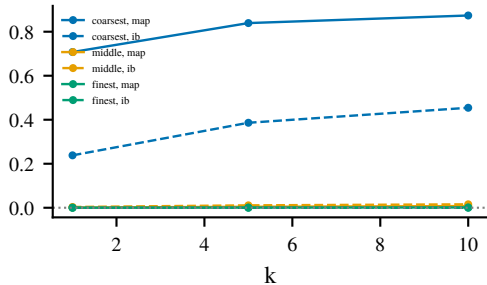
arm c (turn-avg SAE, L19)
