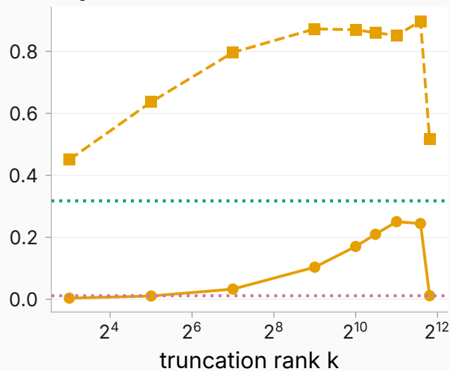
Layer 19
