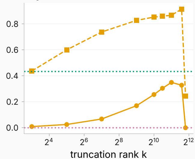
Layer 26
