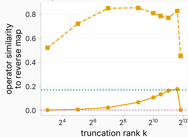
Layer 14
