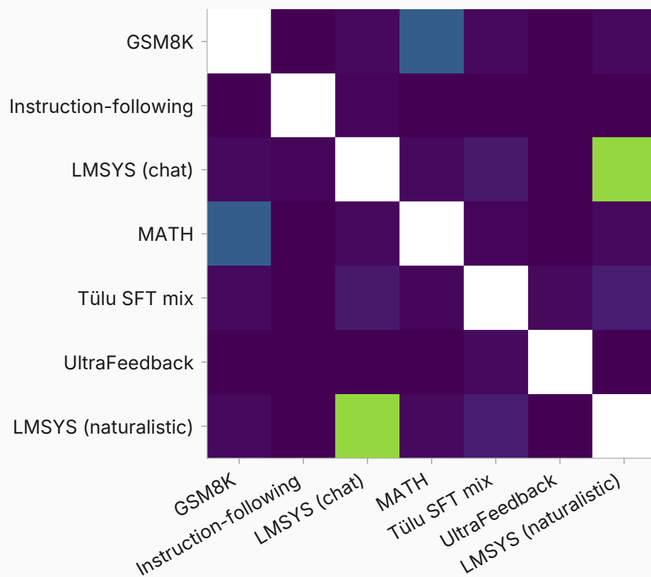
SFT → DPO
