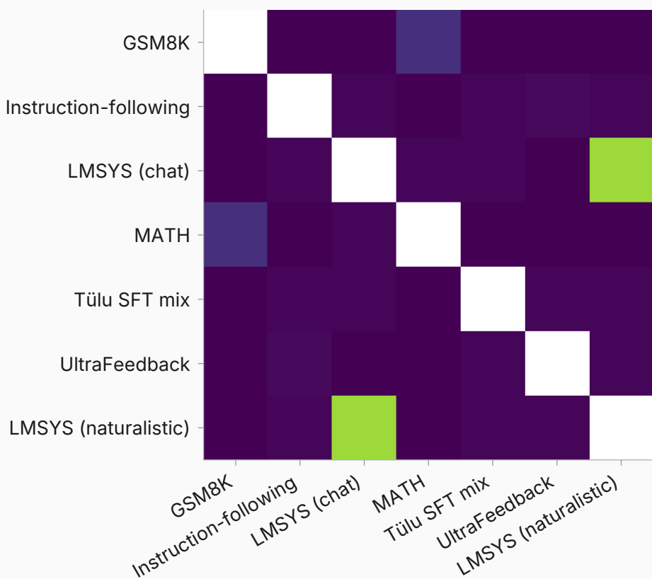
DPO → RLVR
