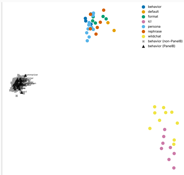
UMAP (n=15, d=0.1, seed 42) — layer 7
