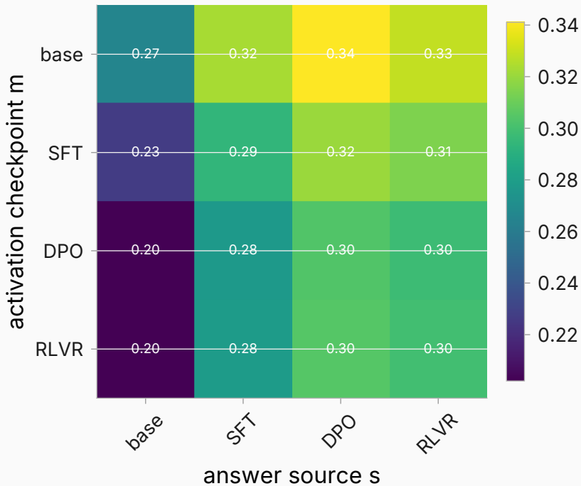
MLP · context arm · single-turn corpus (L31)
