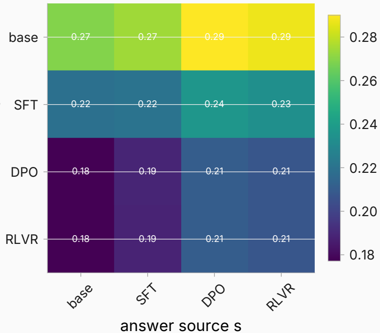
MLP · prefix arm · multi-turn corpus (L31)
