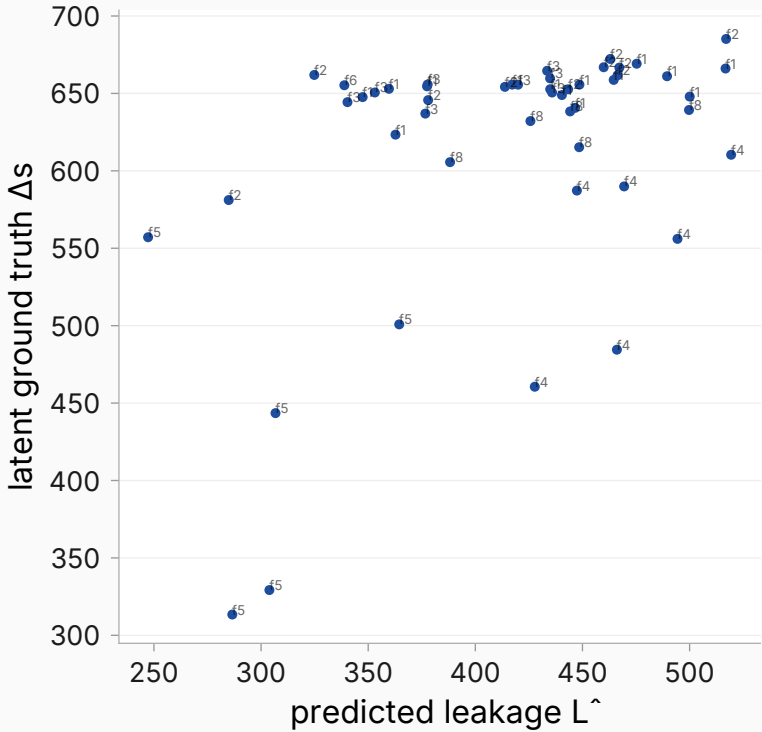
tf_default_posonly_d1_seed42 ( \rho=0.349 )
