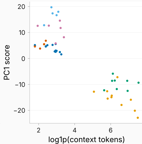
layer 14
