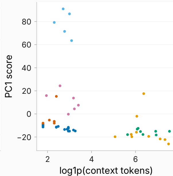
layer 21
