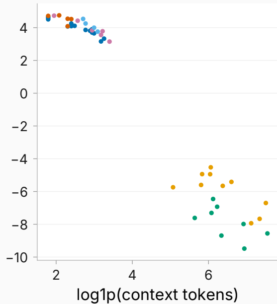
layer 7
