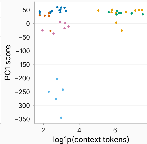
layer 27
