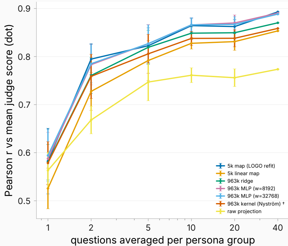
sycophancy (L26)
