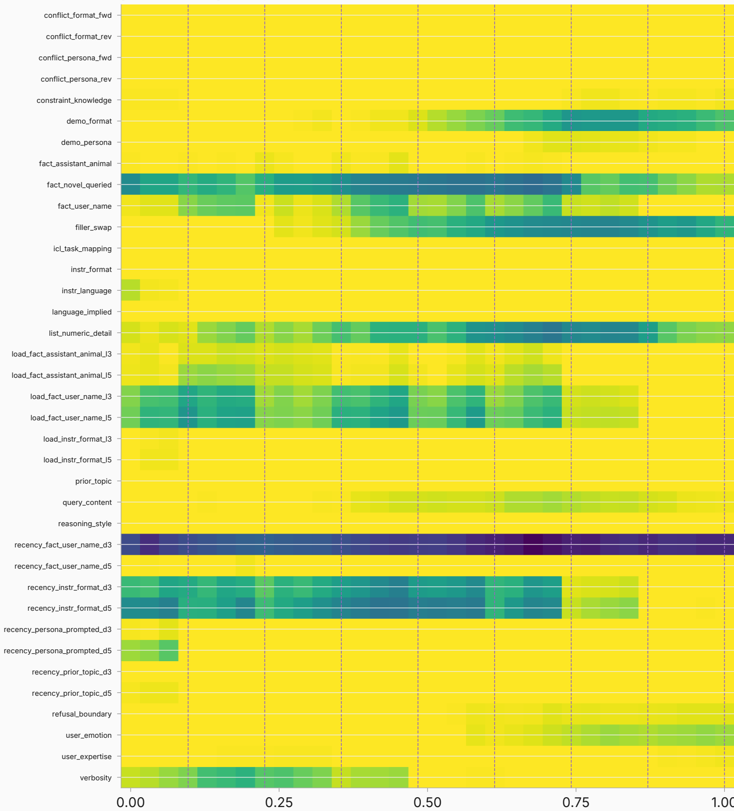
probe AUC per layer — slot ce
