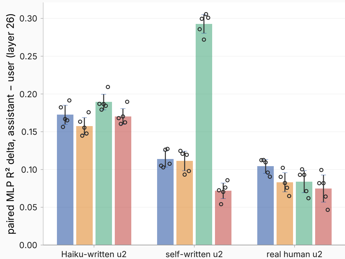
MLP, layer 26 (per-fold deltas, \pm 2SE )
