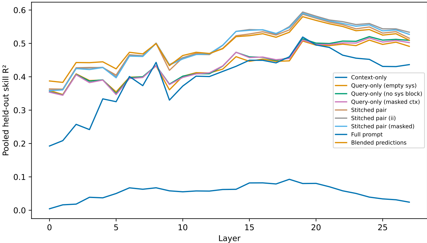
Layer sweep — uc
