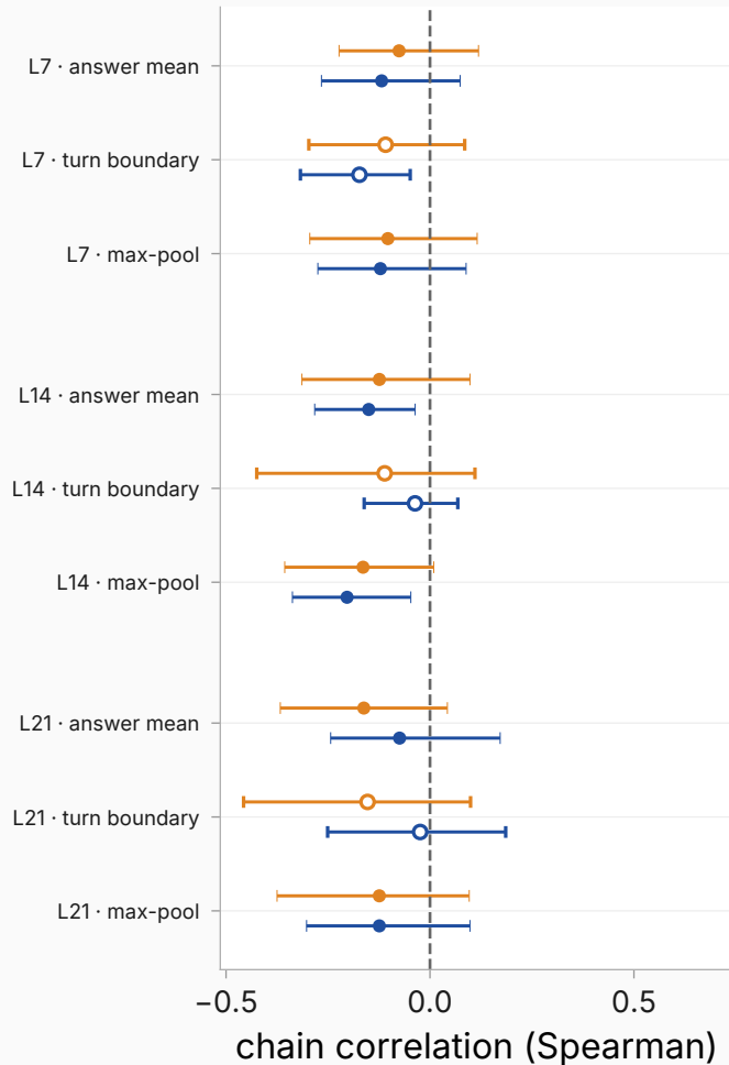
sycophancy
