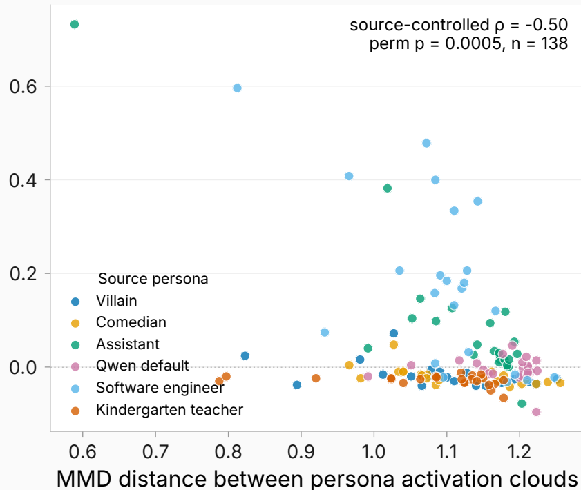
Best cell: MMD, layer 7 (last prompt token)
