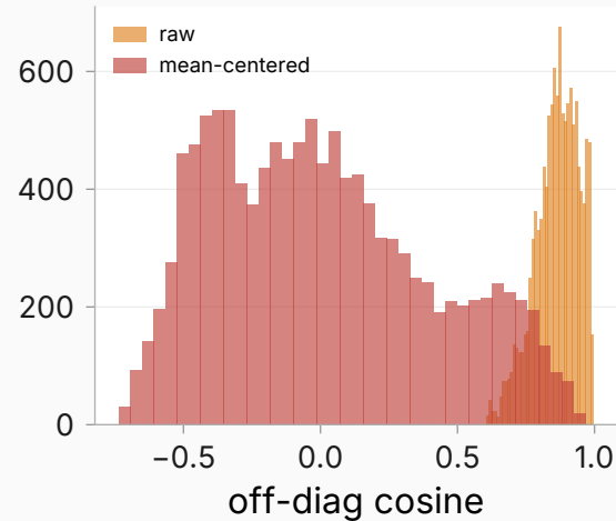
single_token_100p_L20
