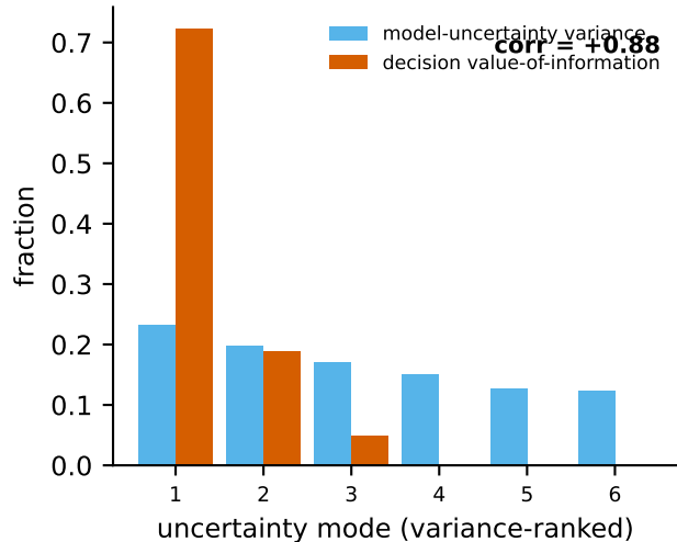
a Chemistry (Buchwald-Hartwig)
