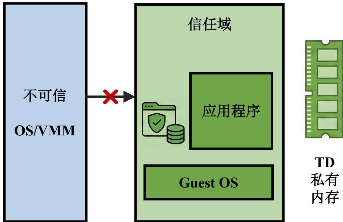
TDX 架构图
