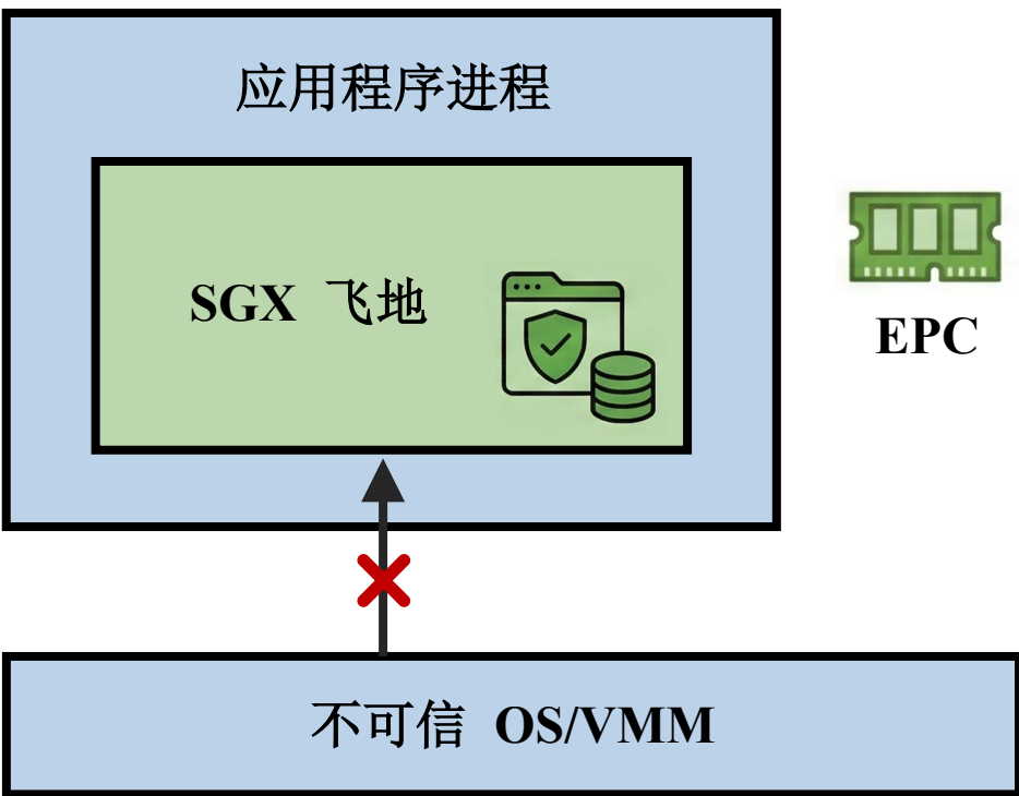
SGX 架构图
