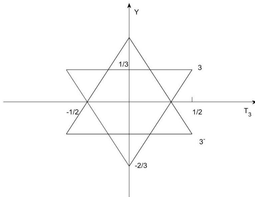
图 5.1 正反夸克多态图
