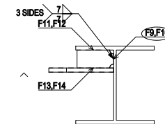
B - E 1:10
