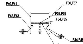
G - G 1:10
