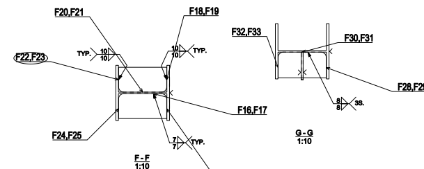
F - F 1:10
