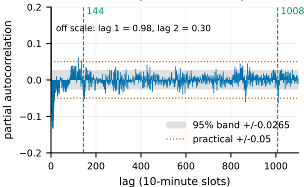
PACF (Levinson-Durbin)
